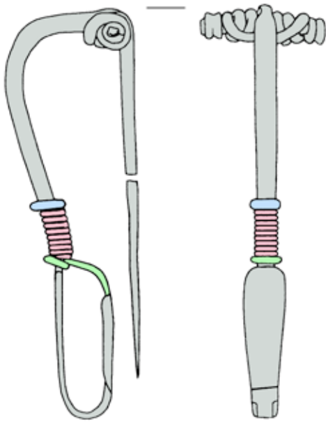
Abb. 4. Schema der Fußkonstruktion. Obr. 4. Konstrukční schéma nožky.
